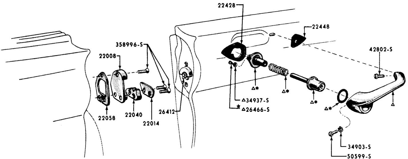
Door Latch/Handle 1959 (Rear)
